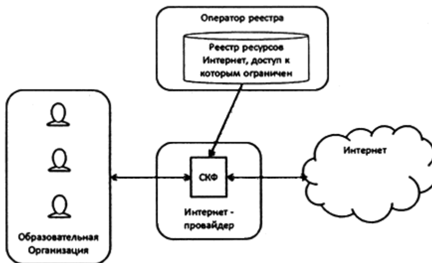
Рис.4. Схема работы контент-фильтрации при размещении у интернет-провайдера
